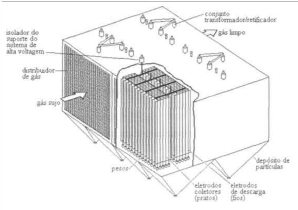
Figura 12 – Precipitador eletrostático
