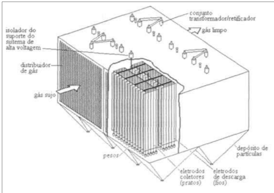
Figura 5 – Precipitador eletrostático
